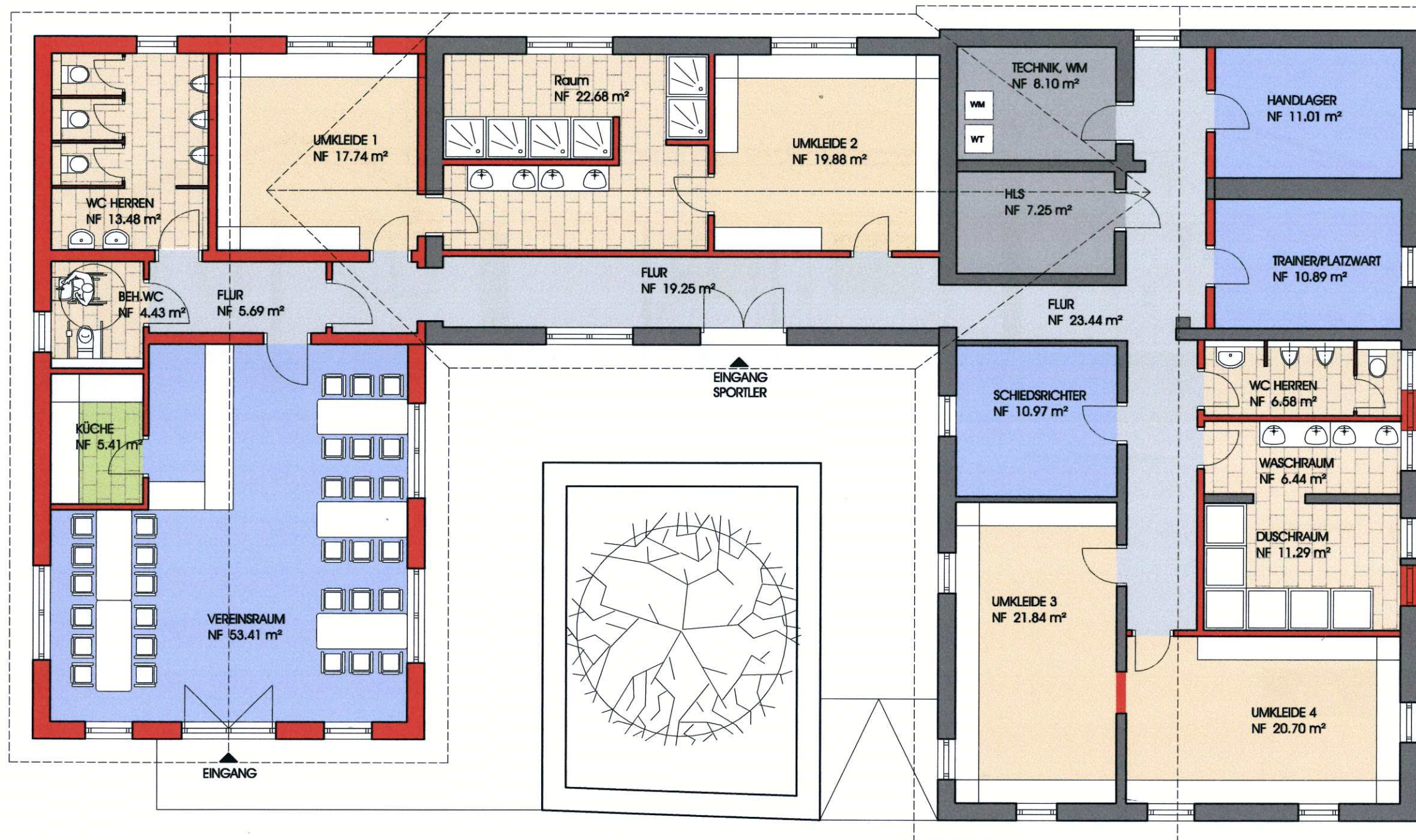
grundriss erdgeschoss
